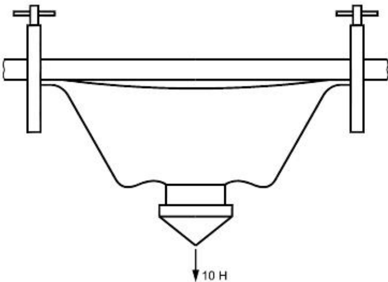
Рисунок 8 - Зажимное устройство для фильтрующей полумаски
