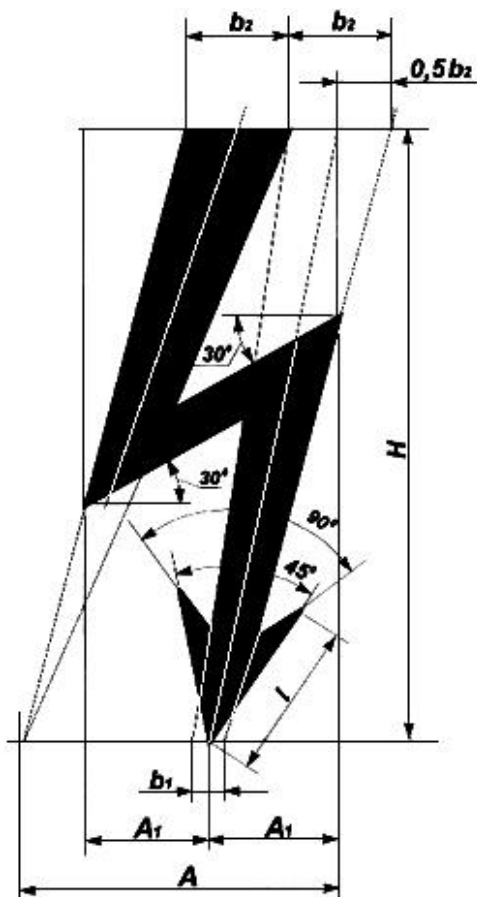
Рисунок Л.1 - Графический символ электрического напряжения
