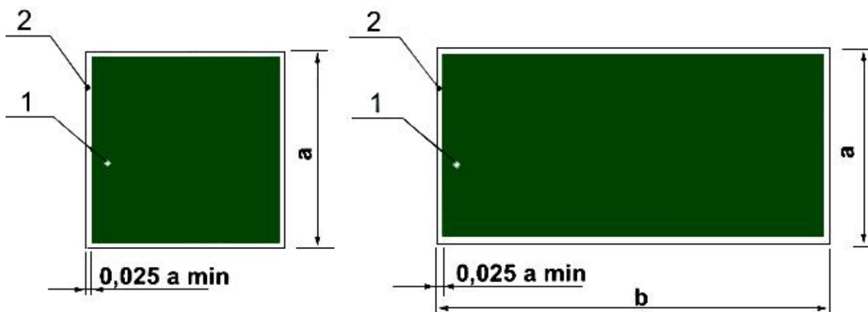
Рисунок 5. Основа цветографического изображения и соотношение размеров эвакуационных знаков безопасности и знаков безопасности медицинского и санитарного назначения
