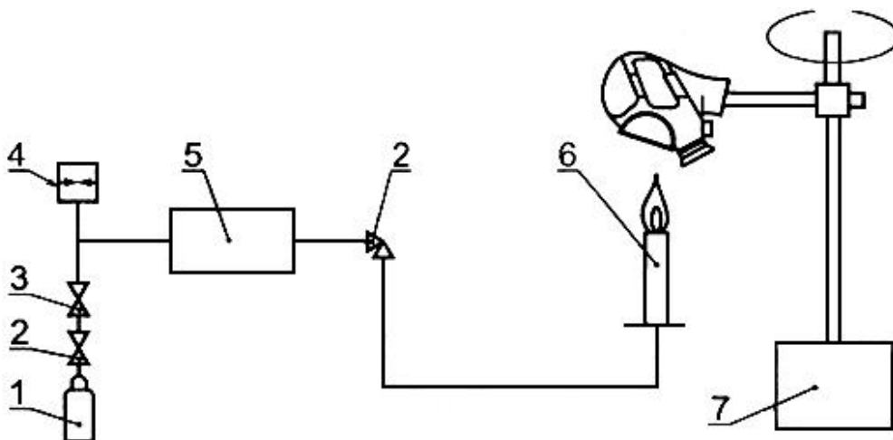
Рисунок 1 - Схема установки для испытания устойчивости к воспламенению масок категории 1
