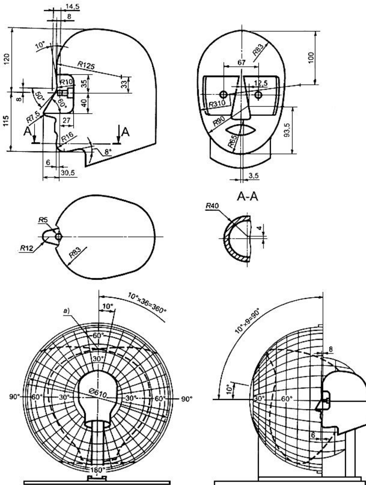
Рисунок 14 - Апертометр
