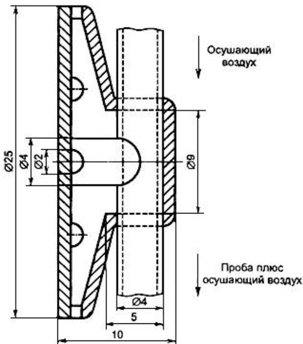
Рисунок 11 - Пробоотборник
