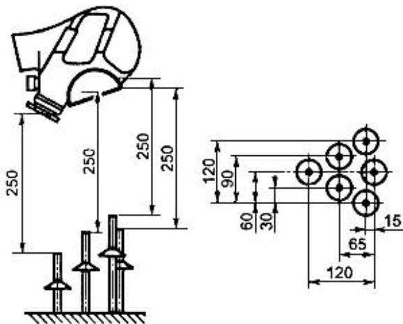
Рисунок 2 - Схема установки, состоящая из шести пропановых горелок
