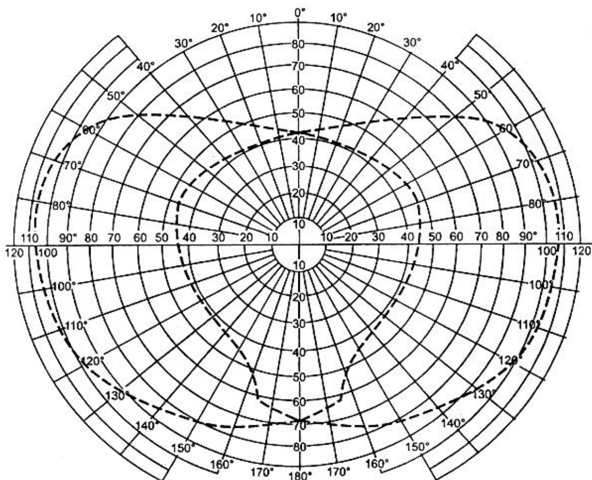
Рисунок 15 - Диаграмма апертометра
