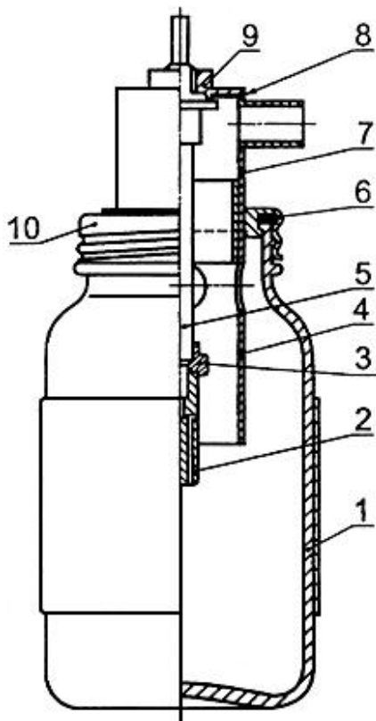
Рисунок 13 - Распылитель
